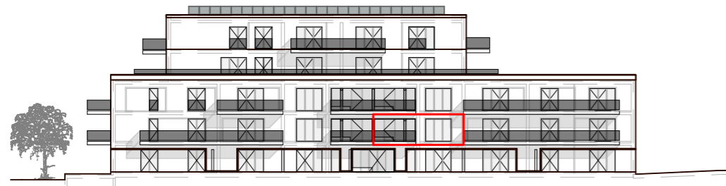
Elévation Sud
