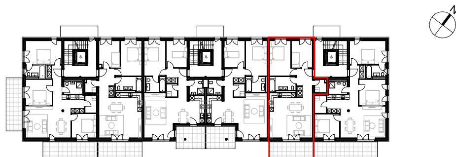
Plan 1 er Etage
