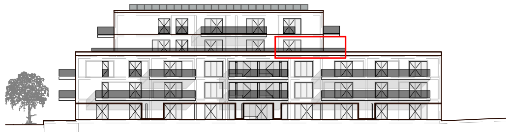
Elévation Sud
