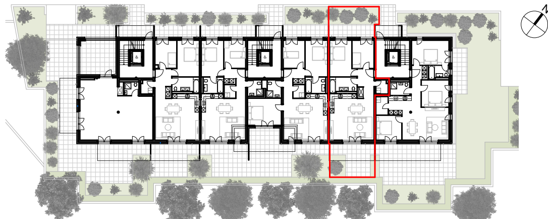
Plan Rez-de-chaussée
