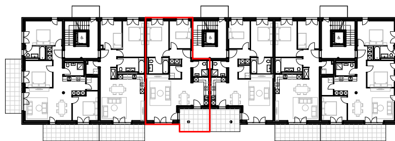
Plan 1 er étage
