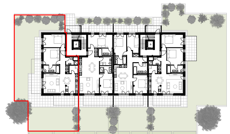
Plan Rez-de-chaussée
