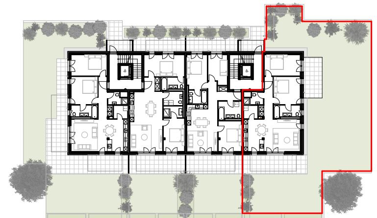
Plan Rez-de-chaussée
